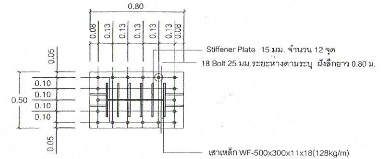
รูปแปลนแผ่นเหล็กยึดเส้าตอม่อกับเส้าเหล็ก
