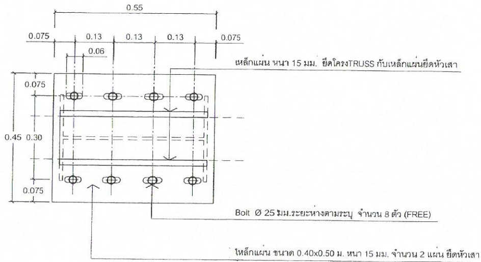
แปลนขยายการยึดโครงTRUSS กับเสาเหล็ก ( FREE )
