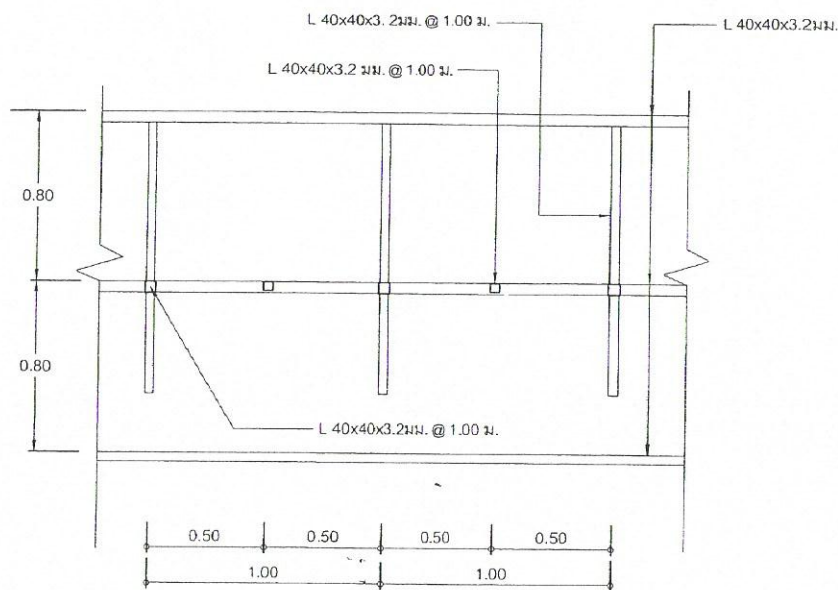
รูปตัด (C) โครงเหล็กงานน้ำฝน มาตราส่วน 1 : 25
