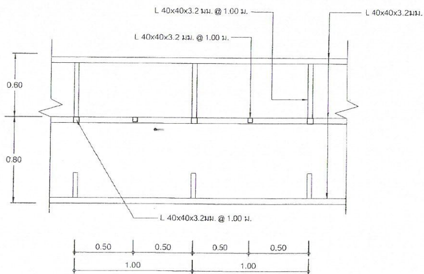
รูปตัด (D) โครงเหล็กงานน้ำฝน มาตราส่วน 1 : 25
