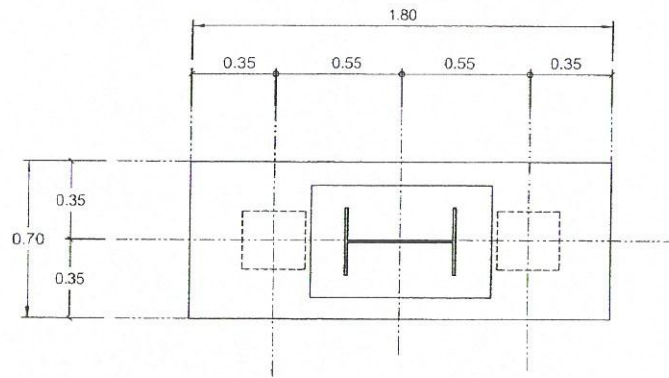
แปลนฐานราก F
