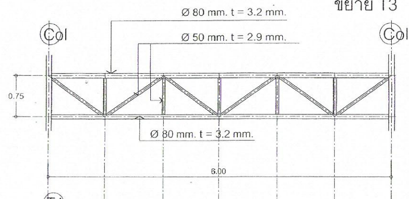
ขยาย T5
