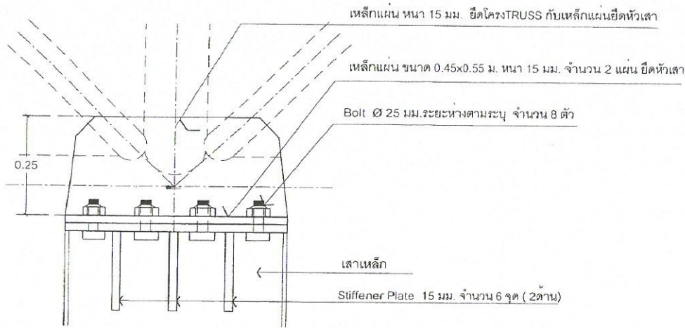
รูปตัดขยายการยึดโครงTRUSS กับเสาเหล็ก
