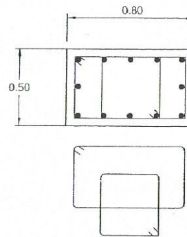
ขยายเส้าตอม่อ C
