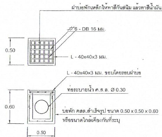
ขยายตะแกรงเหล็ก ฝาบ่อพัก มาตราส่วน 1 : 25
