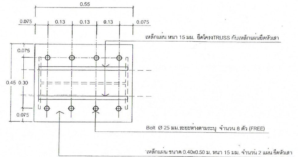
แปลนขยายการยึดโครงTRUSS กับเสาเหล็ก ( FIX )
